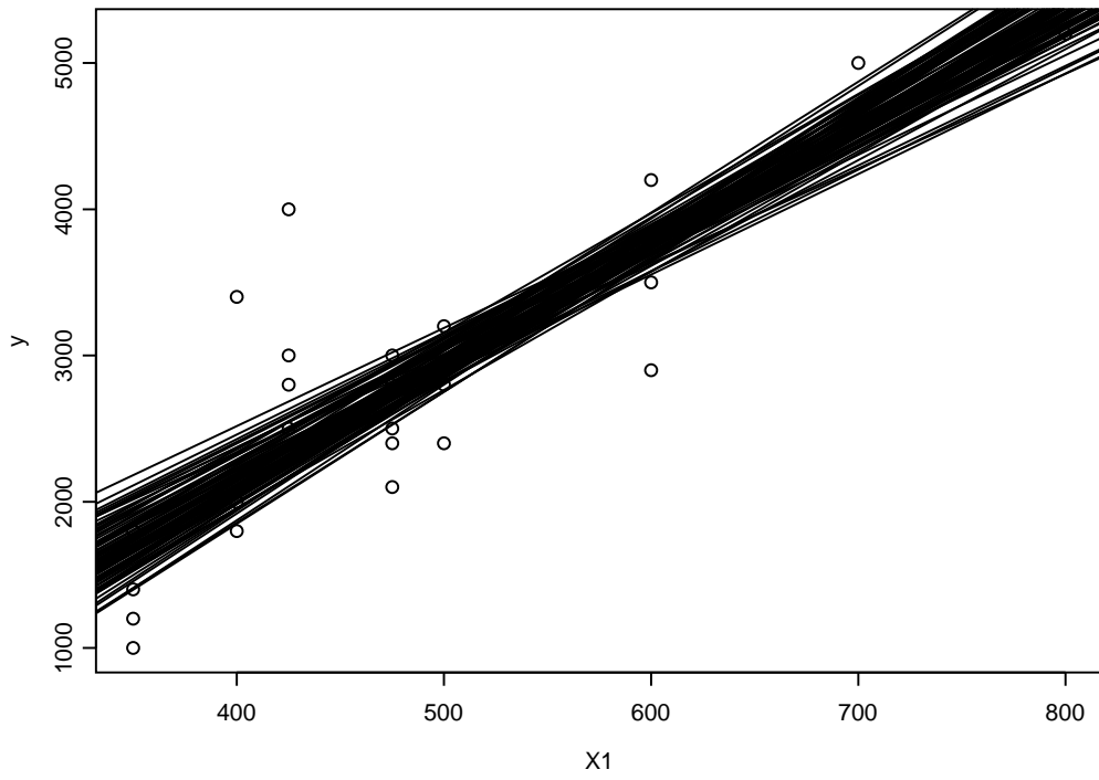
LS bootstrap
