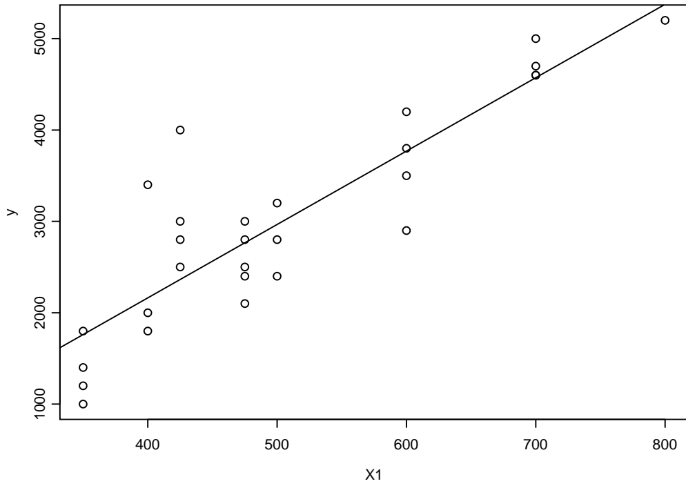
LS fit
